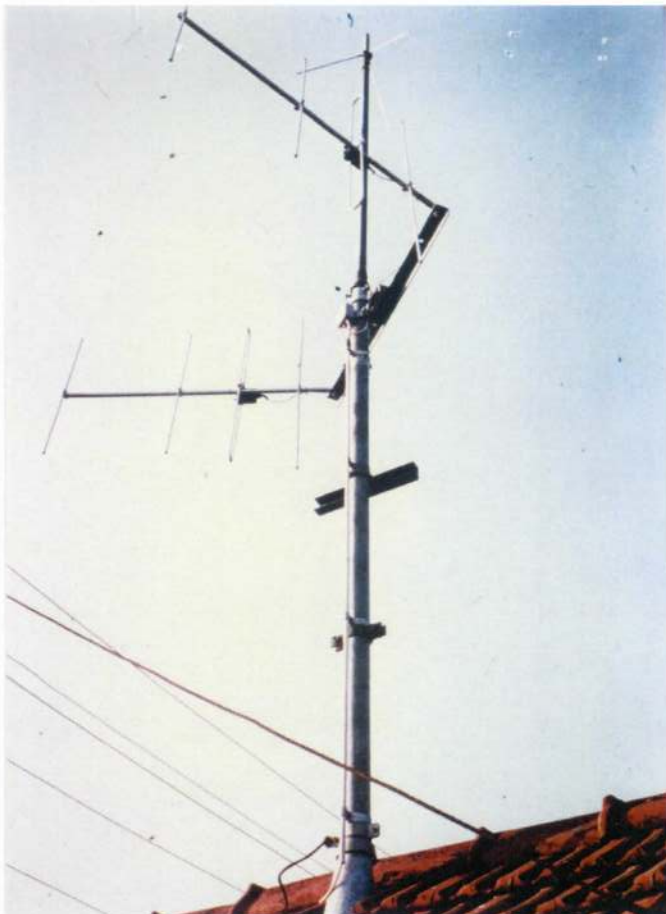
Umbau auf 4 Element Richtantennen
